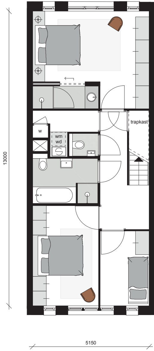
Floris 1e verdieping
